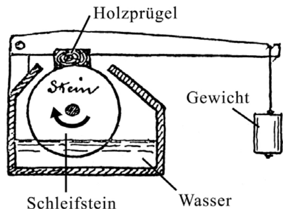
Abb. K 3.17-2 Holzschleifer von Keller (1845)
