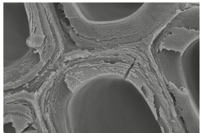
Fichtenholz Tracheiden-Zellwand mit Mikrofibrillen in der Sekundärwand
